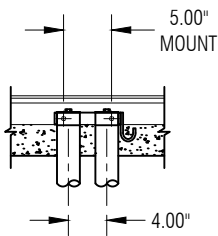
VIEW A-A
